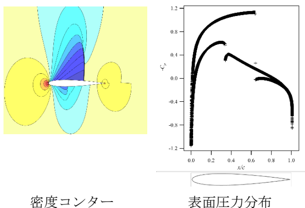
図 8 密度と圧力分布図
