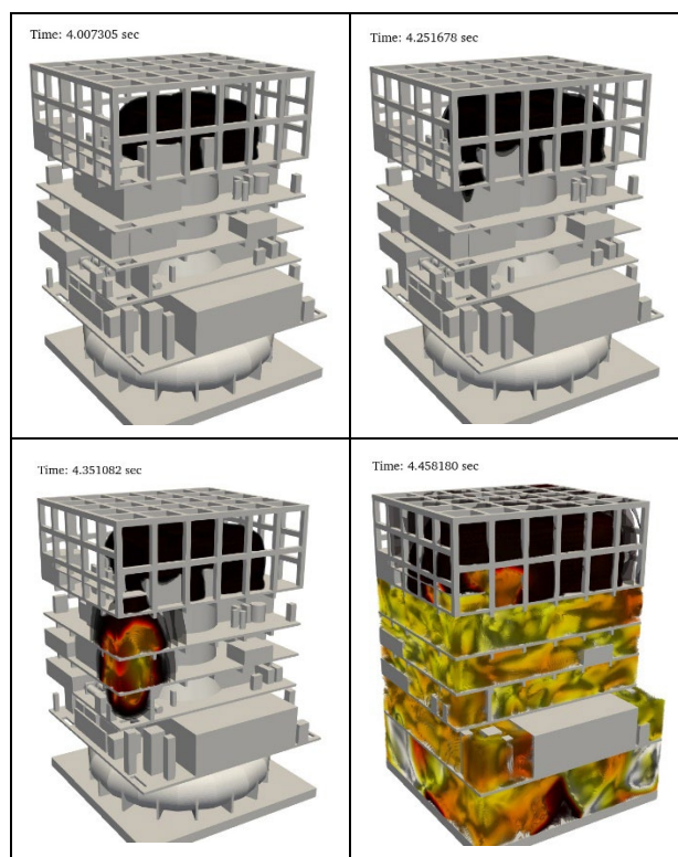
図 34 最上階での着火から乱流燃焼を経て通路3階付近でDDTを生じ、建屋施設内に火炎が伝播する様子
