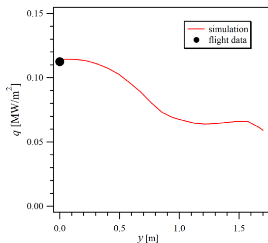
図 29 中心断面上における表面熱流束分布の比較
