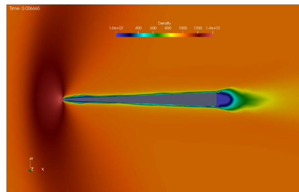
(a) 水流の速度 V=1540\text{m/s} ( \text{Mach}=1.03 )
