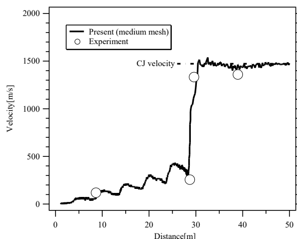
図 31 燃焼波の位置に関する実験との比較
