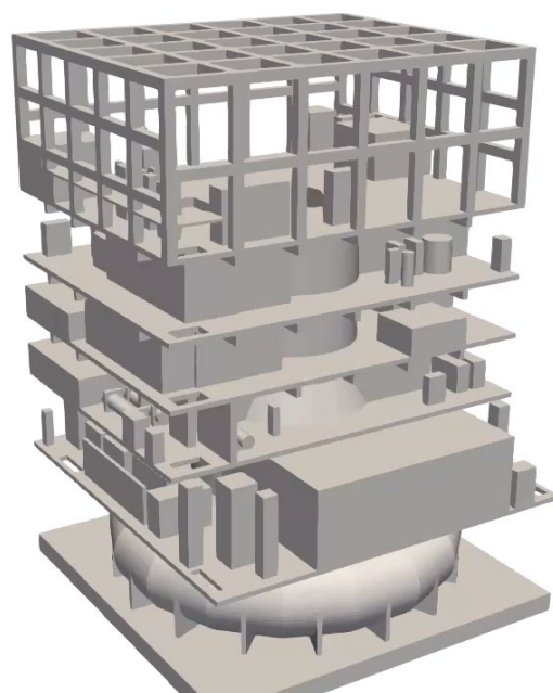
図 33 原子力建屋の形状モデリング例
