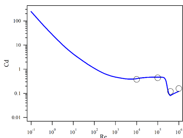
図 23 球に掛かる抗力係数のレイノルズ数効果の再現例
