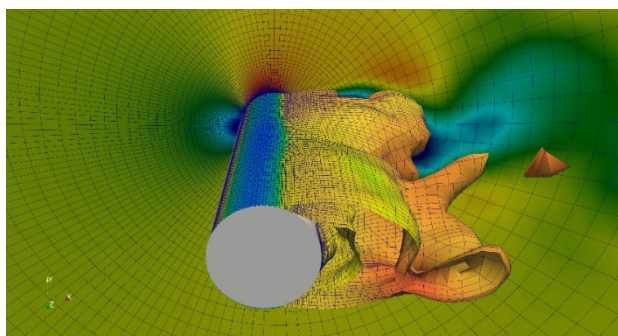
図 21 SST-DDES 機能を用いた Re = 10^6 の場合の解析例、乱流エネルギー k の等値面 (色は圧力情報) と奥行 z = 0 での速度コンター
