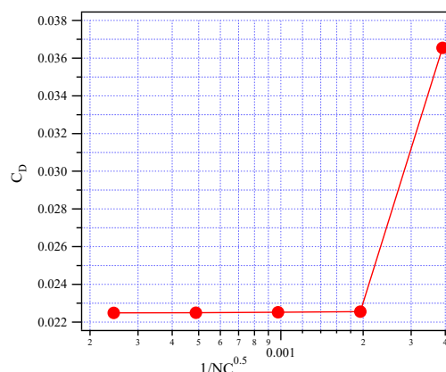
図 10 空力係数の格子依存性
