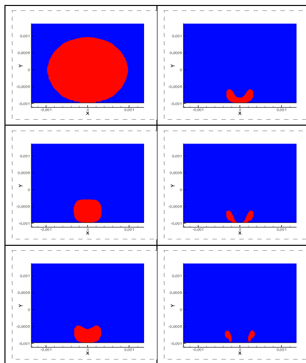
図 40 単一気泡崩壊のシミュレーション例
