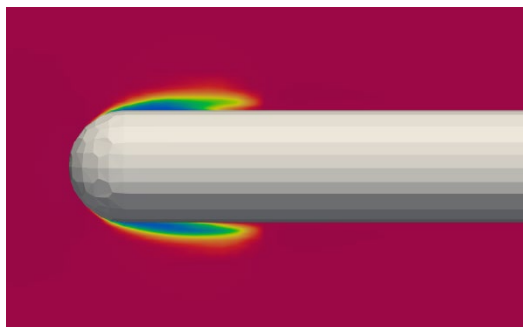
図 36 鈍頭円柱周りに発生するキャビテーションの様子 ( V=4.317\text{m/s} )
