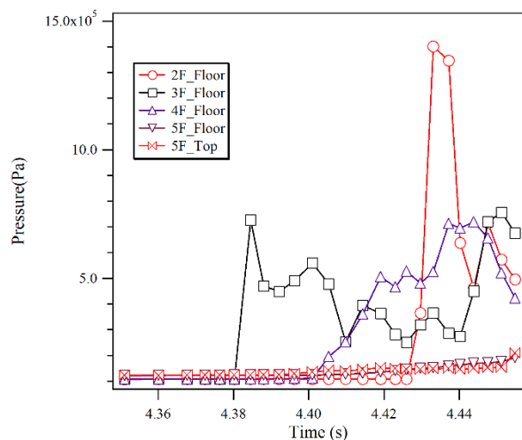
図 35 階段内の各所における圧力の時刻歴
