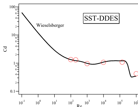
図 18 抗力係数の変化と SST-DDES による再現
