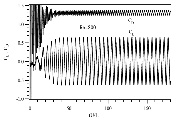
図 16 円柱に作用する抗力と揚力係数( Re=200 )
