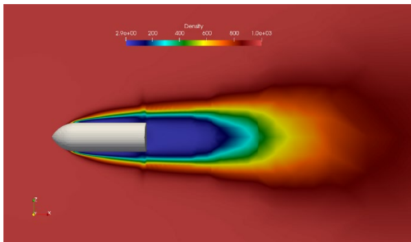
図 38 Ogive 形状周りのスーパーキャビテーション状態の再現例 ( V=102.3\text{m/s} )
