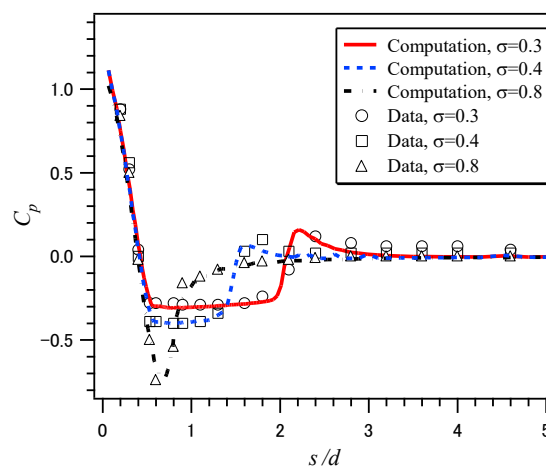
図 37 キャビテーション発生の様子と、実験による表面圧力との比較 ( V=4.317\text{m/s} )
