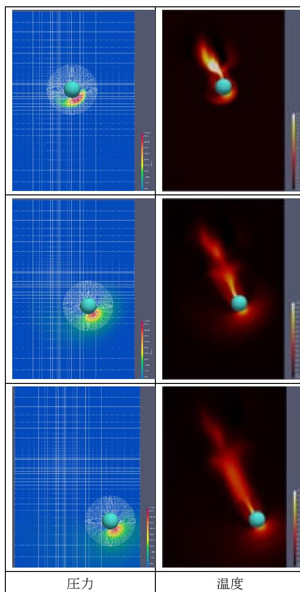
図 43 秒速 1000m/s で水面に突入する球周りに生じる圧力分布と温度分布の様子
