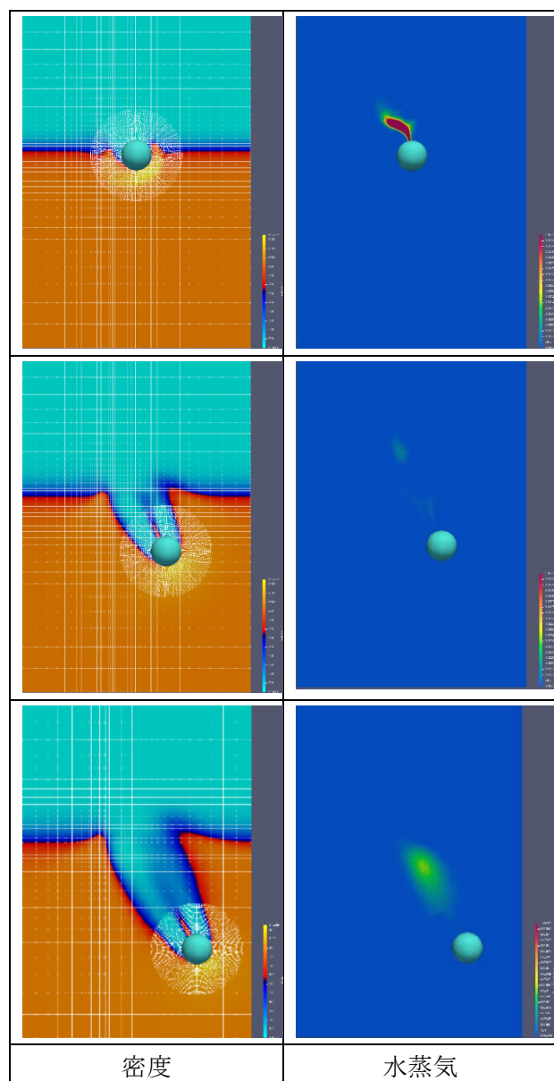
図 42 秒速 1000m/s で水面に突入する球周りに生じるエアレーションとキャビテーションの様子
