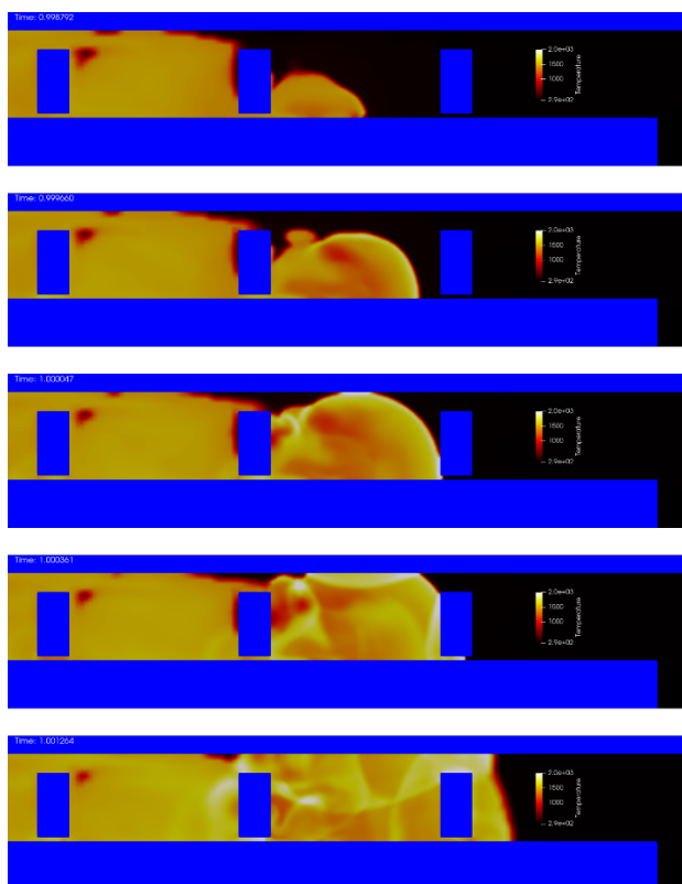
図 32 爆轟へ遷移する時刻の前後における温度場による可視化例
