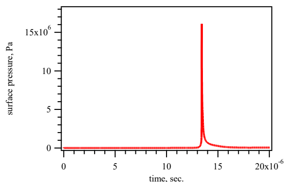
図 41 気泡崩壊に伴う壁面上の衝撃圧の時系列
