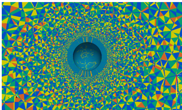
図 22 SST-DDES 機能を用いた球周りの乱流解析に使用した計算格子：マルチカラーによるスレッド分散処理のための色を付けて表示
