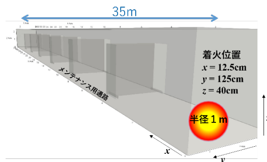
図 30 RUT 施設内を模した計算領域内の配置図
