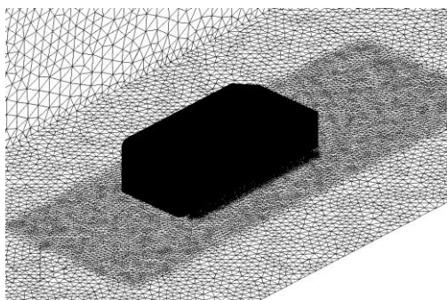
図 2 評価モデル (Ahmed 車体モデル)
