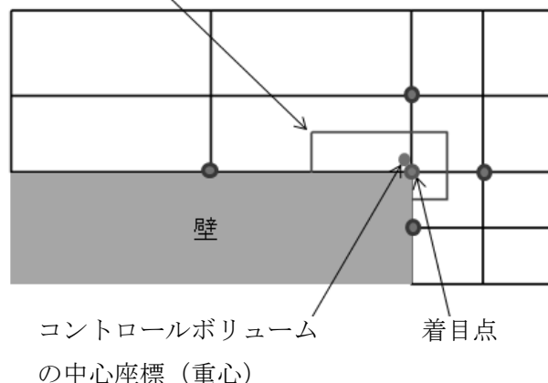
図 9 壁面第 1 格子点の改善
