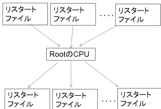
図 12 並列数を変えたリスタート計算機能
