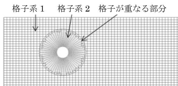
図 4 重合格子
