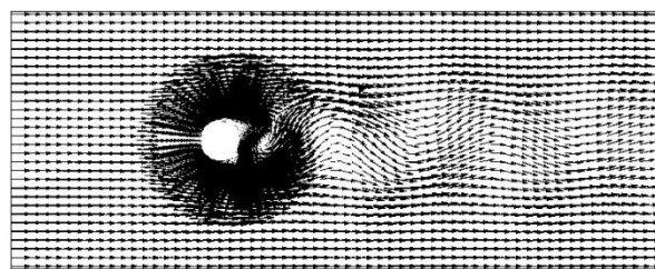
図 5 重合格子による速度分布の計算結果
