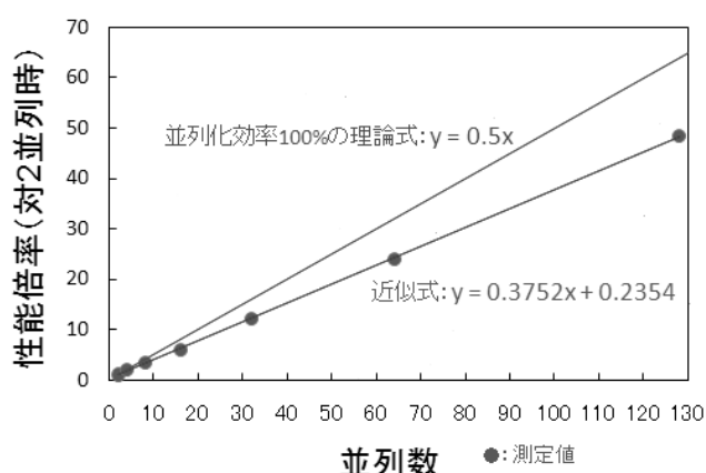
図 3 並列数 2 に対する性能倍率の測定結果
