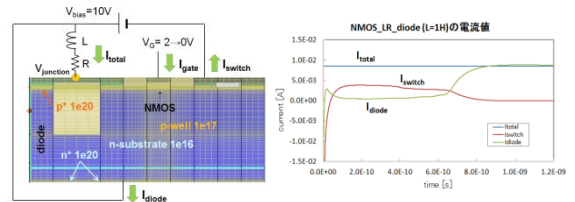
モータ制御回路の解析事例
