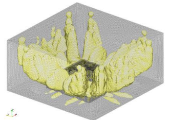
屋外環境騒音解析
